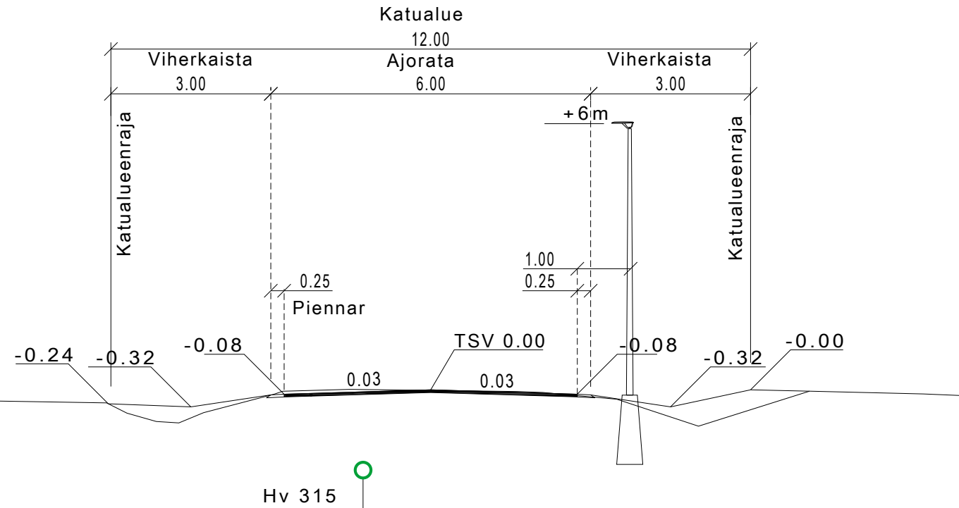
Tyypipoikkileikkaus Laiduntie (pl 80)
