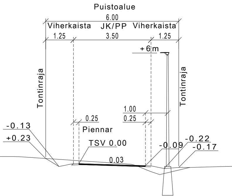
Tyypipoikkileikkaus Laiduntie (pl 300)
