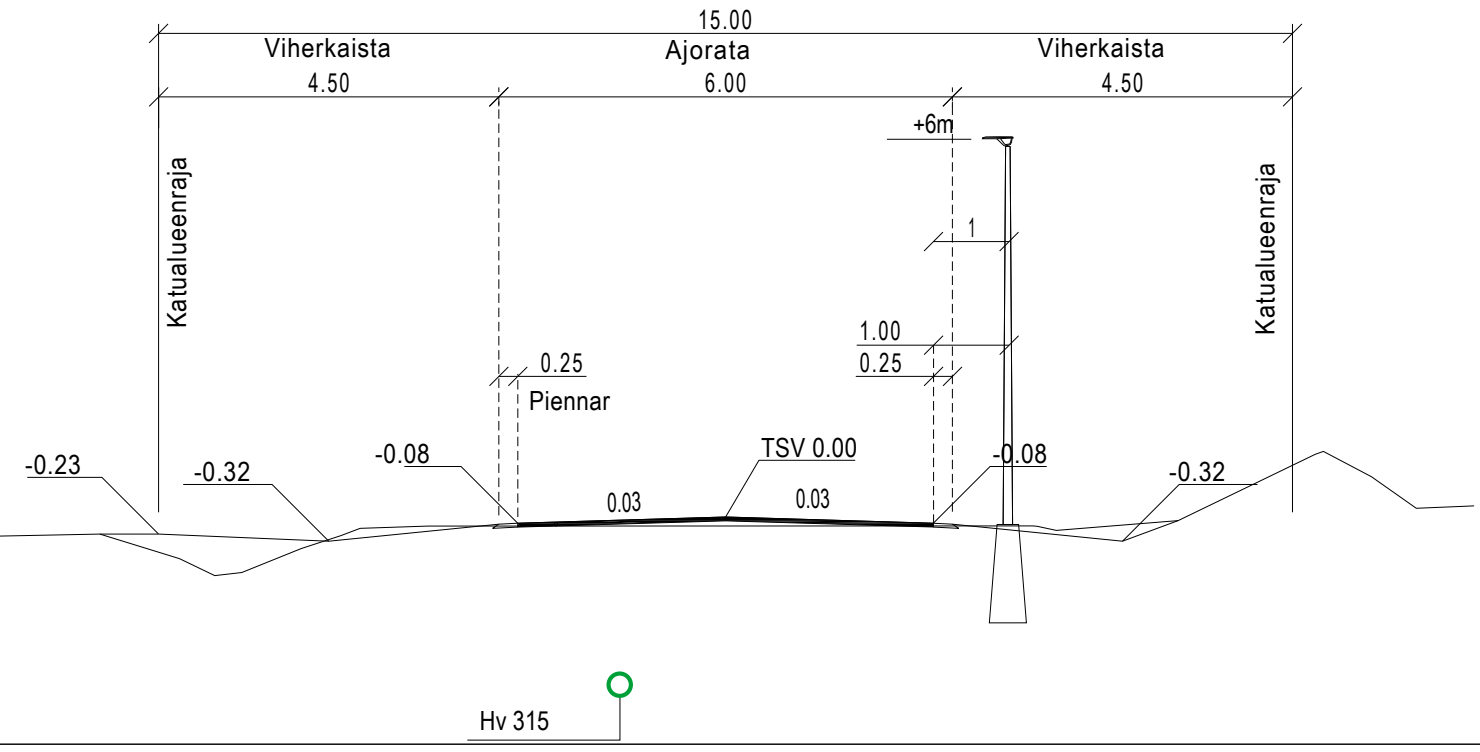
Tyyppipoikkileikkaus Pajupurontietie (pl 500)
