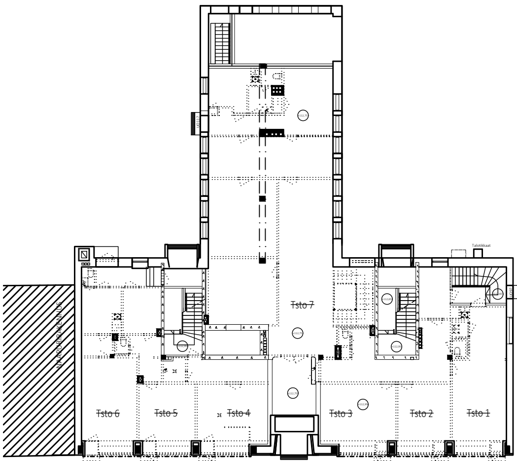
Purettavat 1:250
