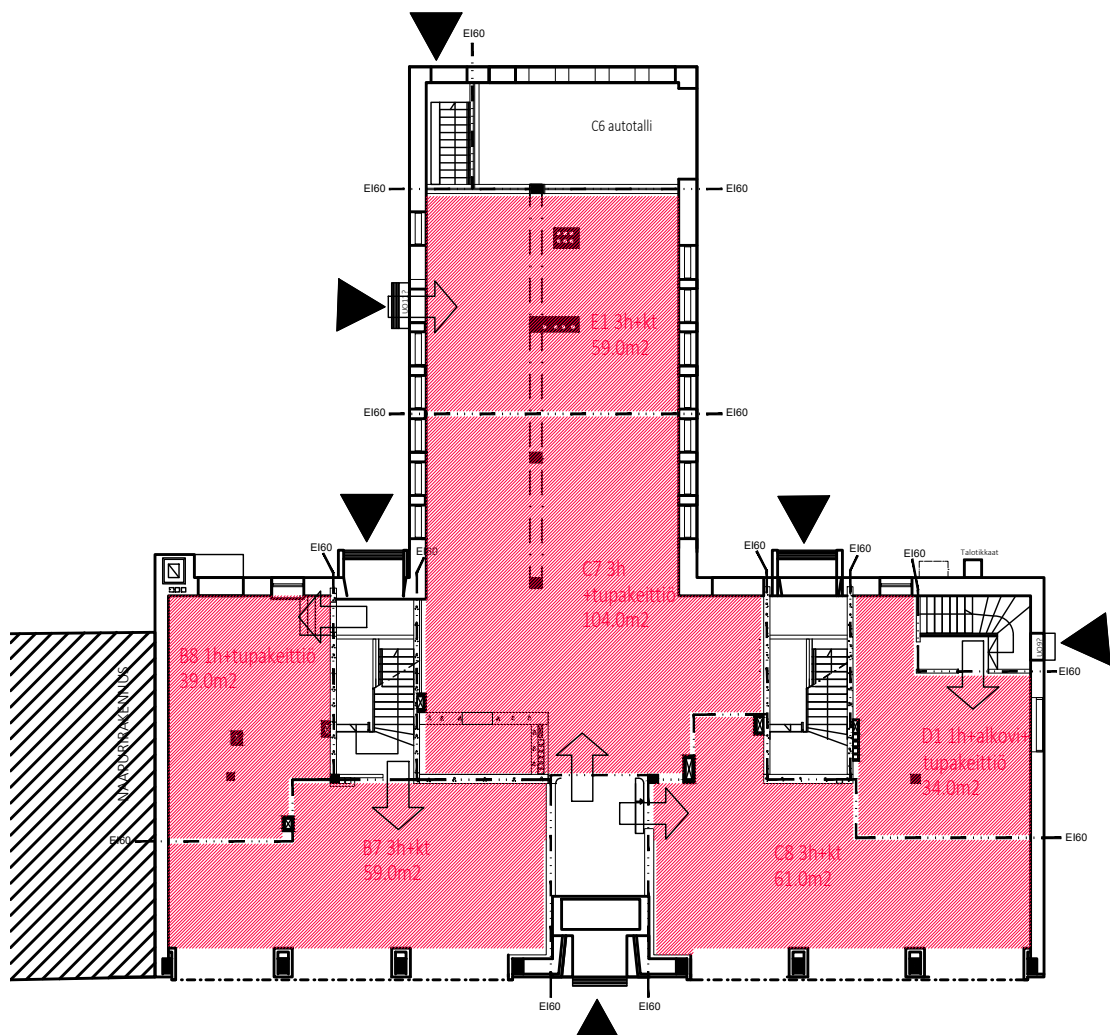
Huoneistojako ja muutosalueet 1:250
