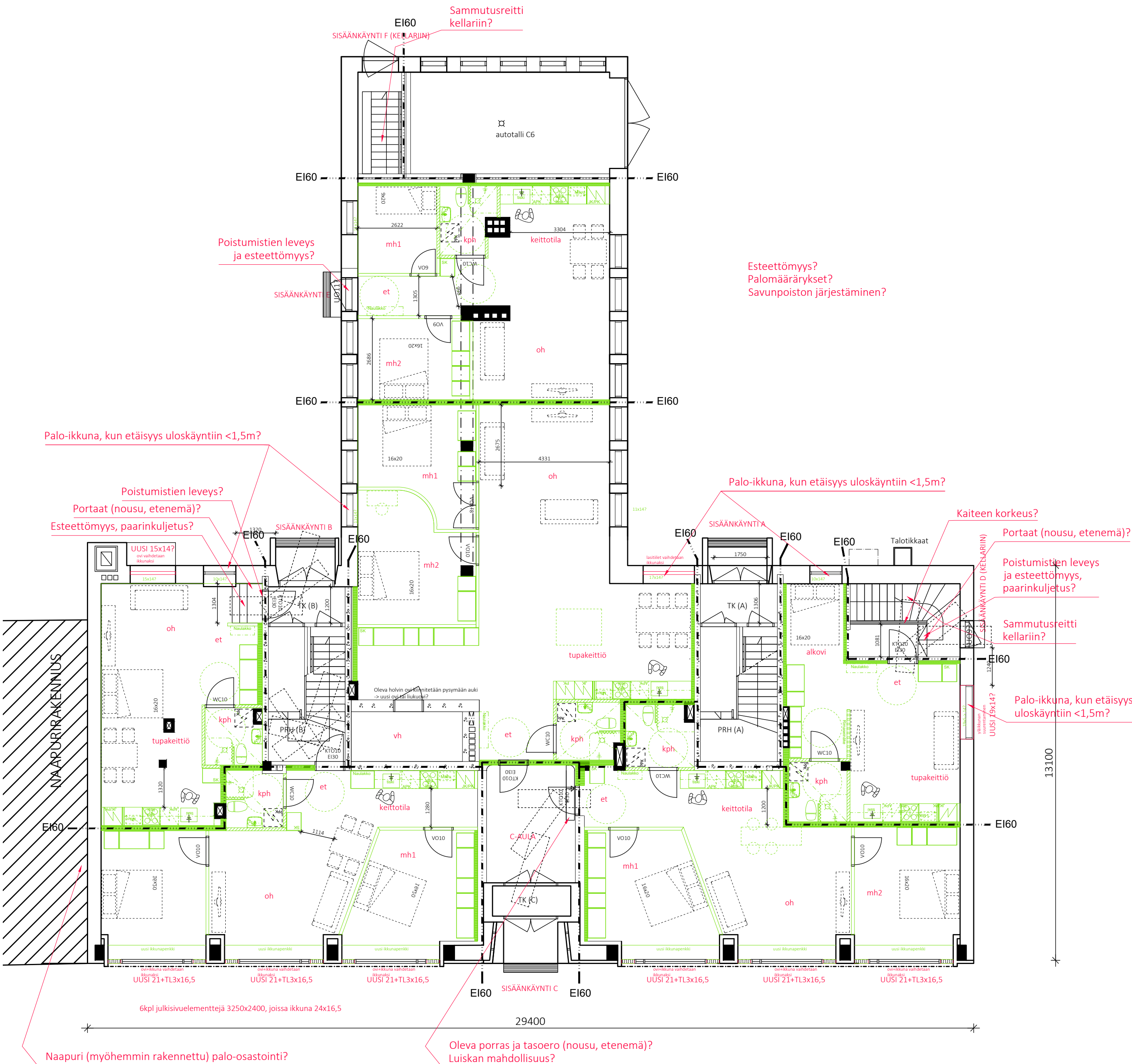
Pohjapiirustus 1:100
