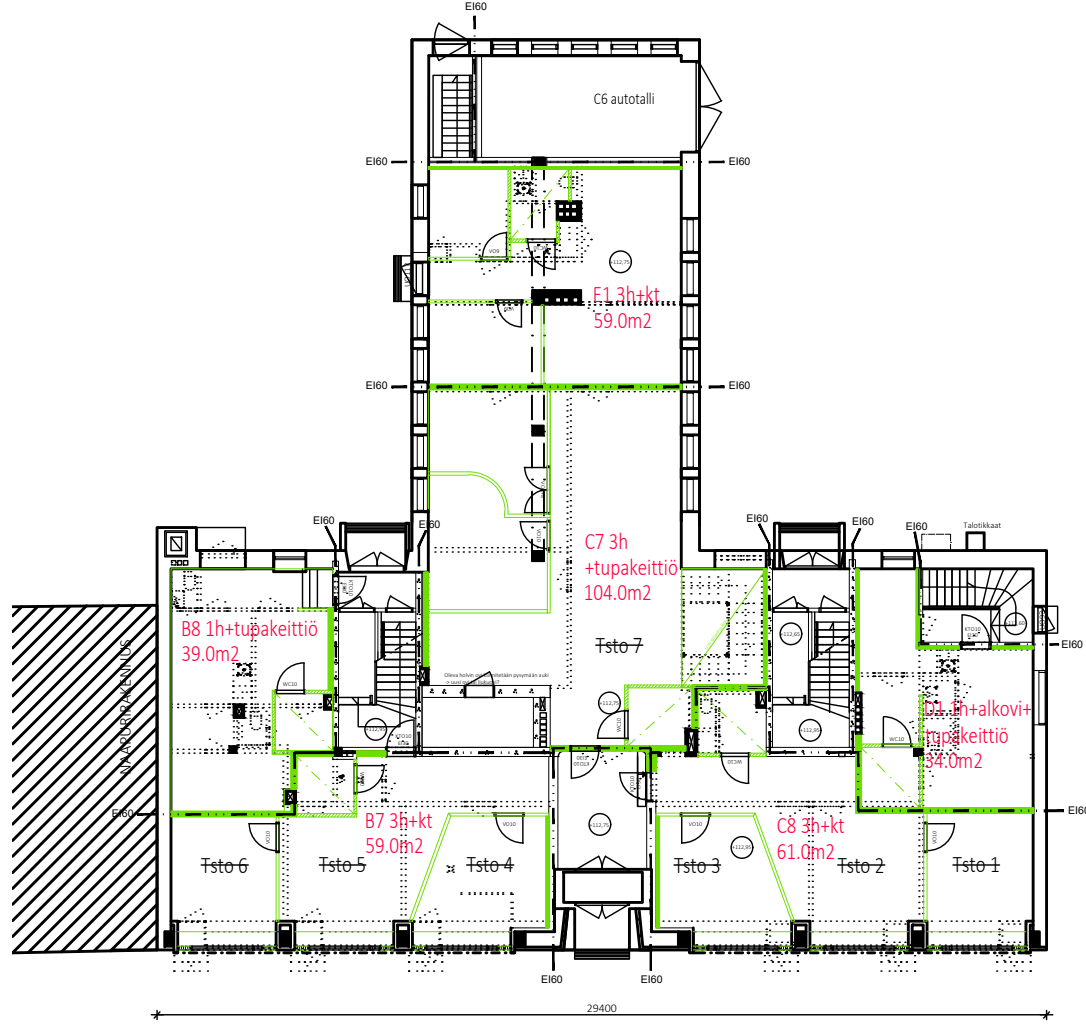
Huoneisto- ja huonejako + purettavat 1:250
